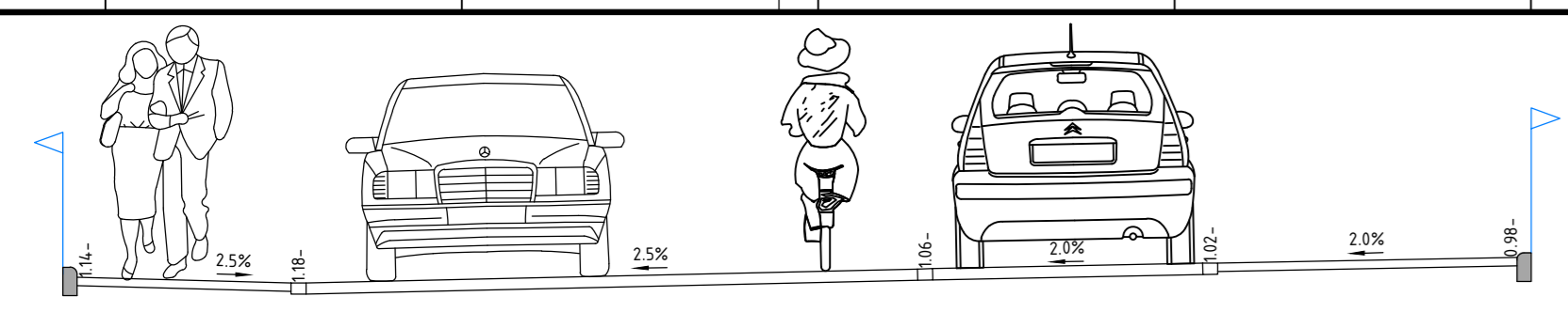
Dwarsprofiel B-B Overlaat Schaal 1:50
