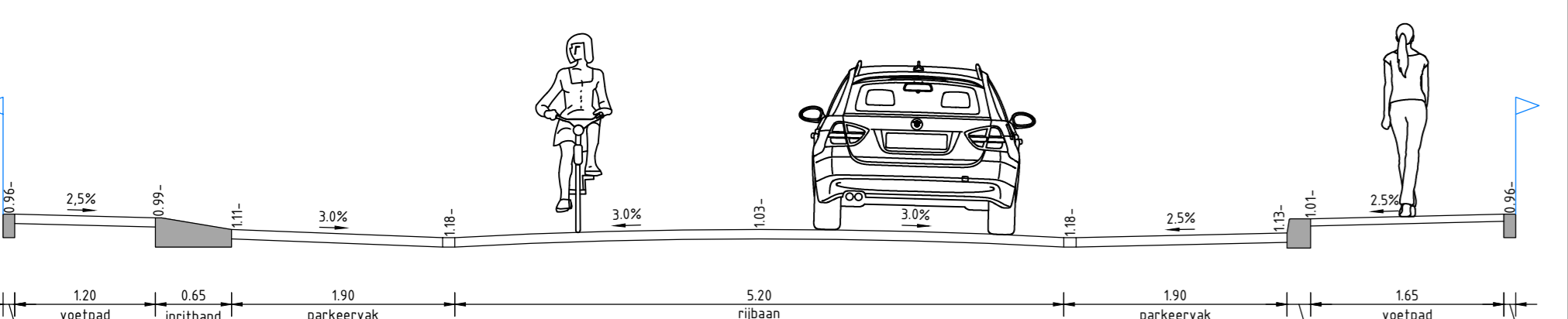
Dwarsprofiel A-A Hoepel Schaal 1:50
