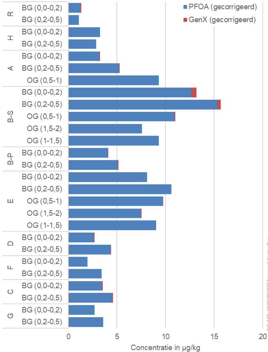
Figuur 18 PFOA- en GenX-concentraties in de diepte (gecorrigeerd, exclusief de resultaten uit de kas uit cluster B-S). PFOA-concentraties in de buurt van de fabriek zijn het hoogst zijn in laag II. Dit wijst er op dat de atmosferische depositie van PFOA gestopt is en er uitspoeling plaatsvindt. Diepte lagen: I = 0 - 0,2 m-mv; II = 0,2 - 0,5 m-mv; III = 0,5 - 1 m-mv, IV= 1 - 1,5 m-mv; V= 1,5 - 2 m-mv
